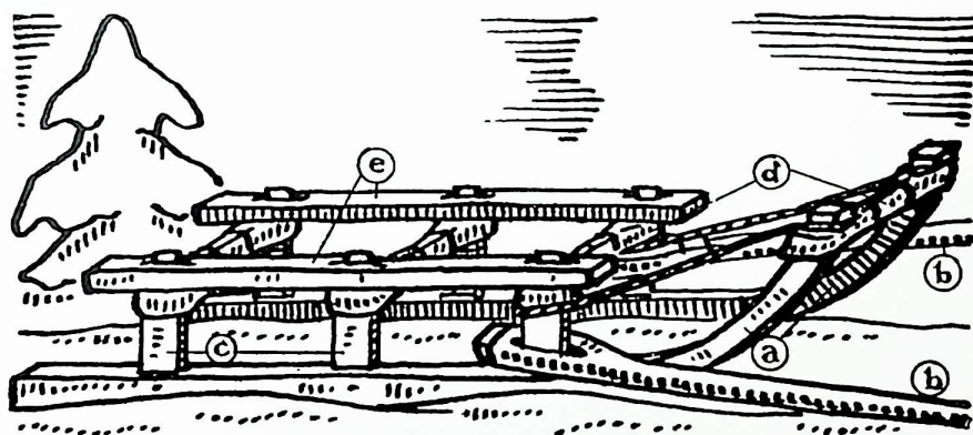
Ragavas. a – Slieces, b – ilksis, c – mietnes, d – balzieni, e – uzkalas.
