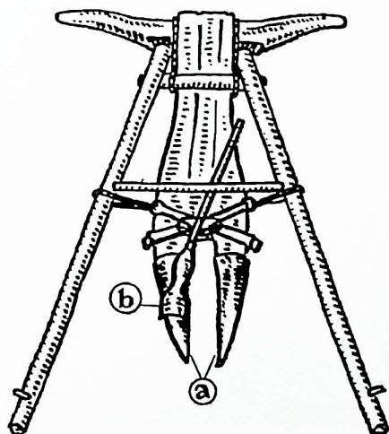
Spīļu arkls; a – lemeši; b – vērstuve (ar spīļu arklu arot, vērstuvi uzliek vai nu uz viena vai otra lemeša atkarā no tā, uz kuŗu pusi vēlas, lai velēna kristu.
